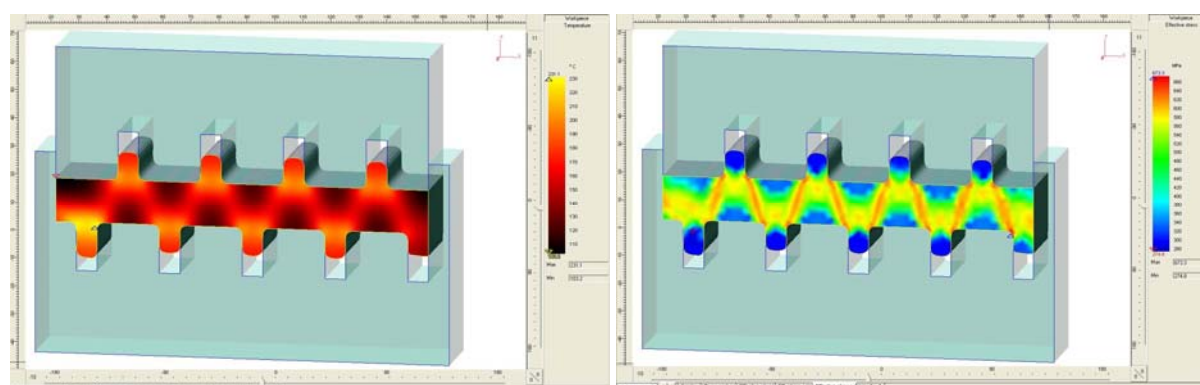
а) Разпределение на температурата в обема на заготовката б) Разпределение на интензивността на напреженията
