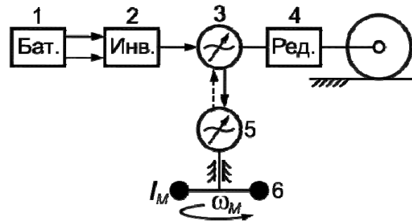
Фиг. 9 Структурна модификация на електромобил, включваща електрическа батерия 1, инвертор 2, асинхронни честотно управляеми мотор-генератори 3 и 5, зъбен редуктор 4 и маховик 6
