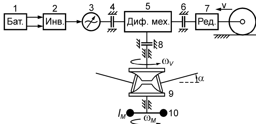
Фиг. 10 Структурна модификация на електромобил, включваща електрическа батерия 1, инвертор 2, честотно управляеми асинхронни електродвигател 3, съединители-спирачки 4, 6 и 8, диференциален планетен механизъм 5, зъбен редуктор 7 и фриксионен вариатор 9 и маховик 10
