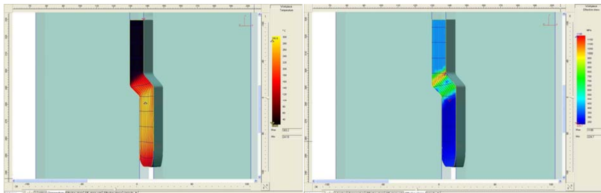
а) Разпределение на температурата в обема на екструдирания заготовка б) Разпределение на интензивността на напреженията
